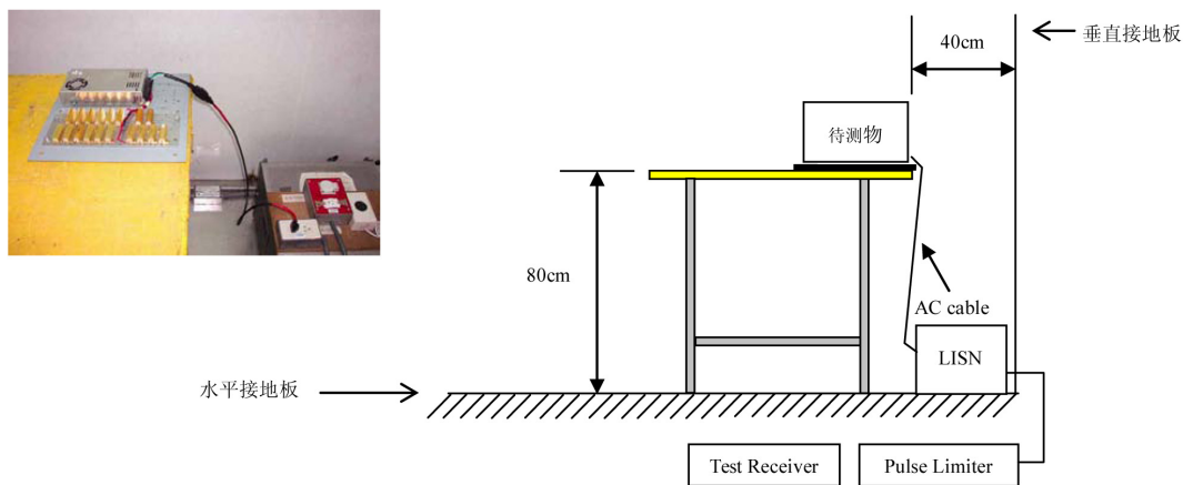
圖一 昂鼎 EMI 測試系統配置圖
