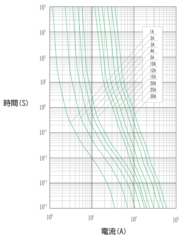
時間-電流曲線
