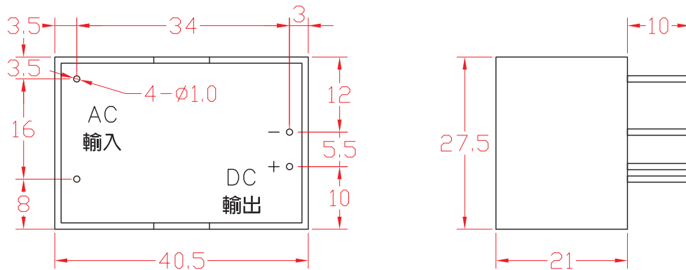
底視圖
