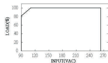
降額曲線
